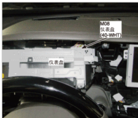
62.仪表板左侧
