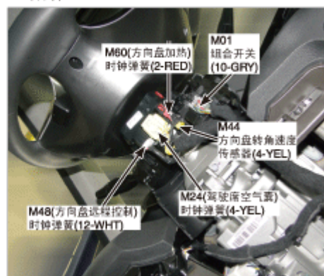
66.转向柱
